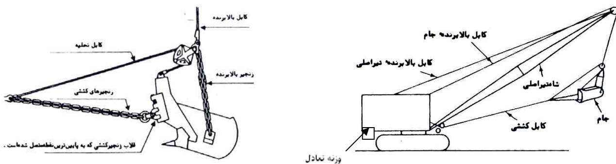
شکل شماره ۲-۱۲-۲- قسمت های اصلی دراگلاین
