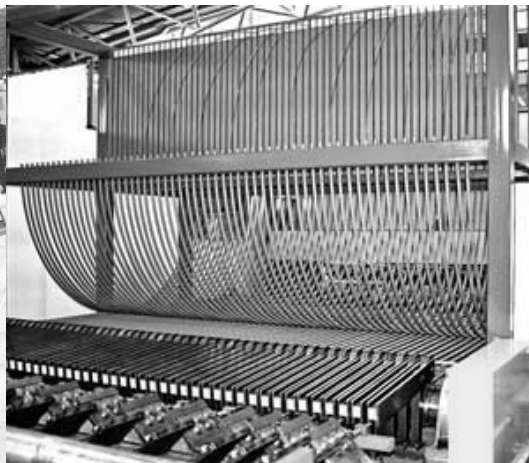
شکل ۴-۱۲-۱۲- نمایی از ماشین آلات مورد استفاده در خط تولید شبکه های میلگرد
