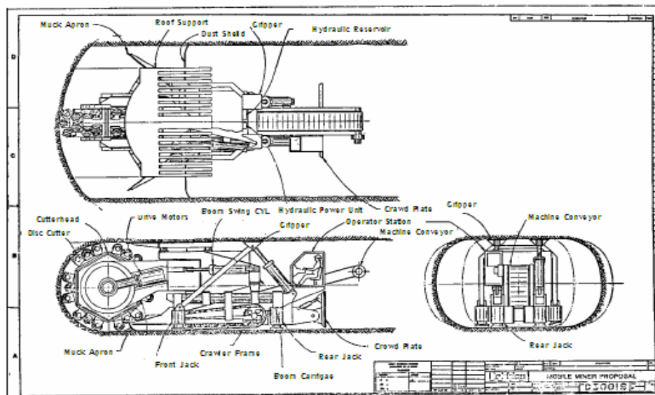
شکل ۳-۲۳-۷- نمایش قسمتهای اصلی ماشین
