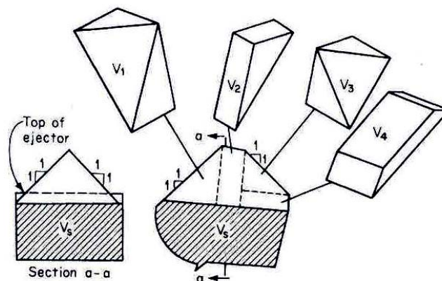
شکل ۲-۶-۵- ظرفیت پر و انباشته اسکرپر
