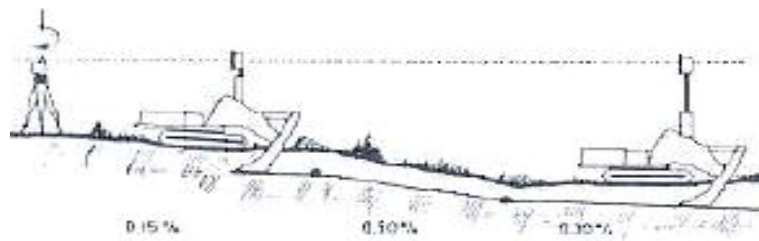
شکل شماره ۵-۷-۵- فرستنده اشعه لیزر
