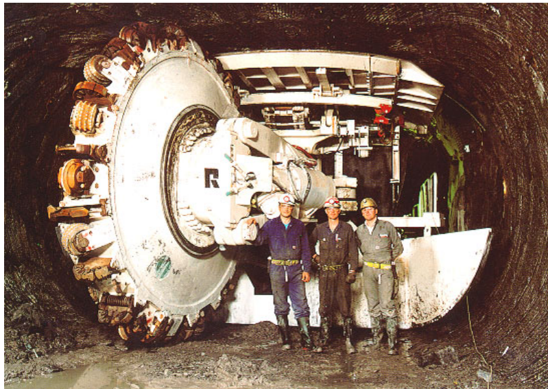
شکل ۳-۲۳-۱- نمایی از یک Mobile Mine در تونل
