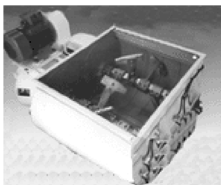
شکل شماره ۴-۳-۸- نمونه میکسر افقی
