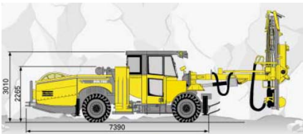
شکل ۳-۲-۱، Bolter ساخت اطلس کوپکو
