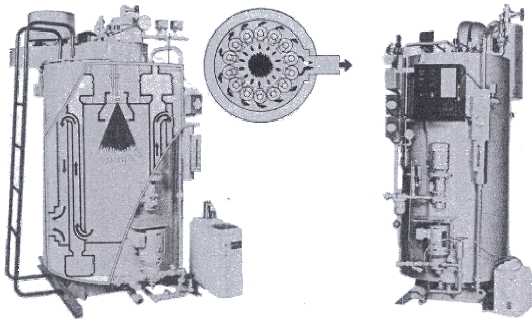
شکل ۴-۷-۳- دیگ بخار
