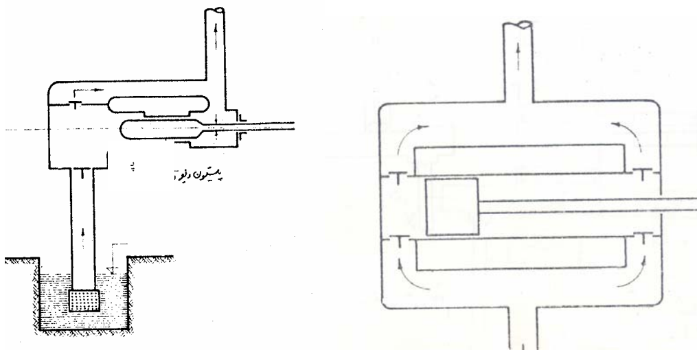
پمپ رفت و برگشتی پلانجر
