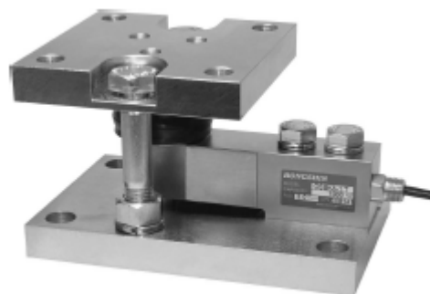
شکل شماره ۴-۵-۱- سلول فشاری
