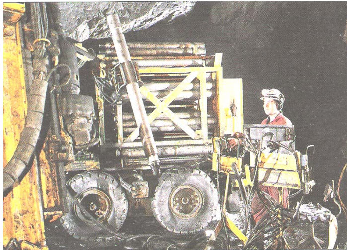
شکل ۳-۱۸-۵- نمایش سیستم جایجایی اتوماتیک لوله‌های حفاری
