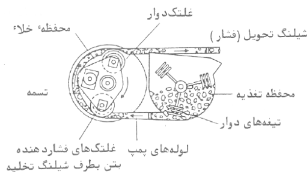
شکل ۴-۱۰-۸- قسمتهای اصلی پمپ بتن
