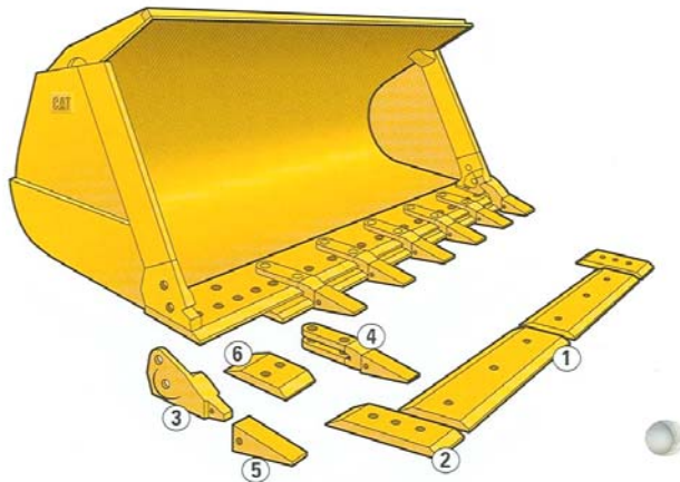
شکل شماره ۲-۱-۵- جام حفاری عمومی
