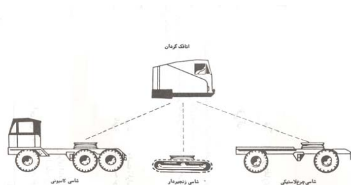
شکل ۴-۷-۱- تقسیم بندی انواع جرثقیل متحرک
