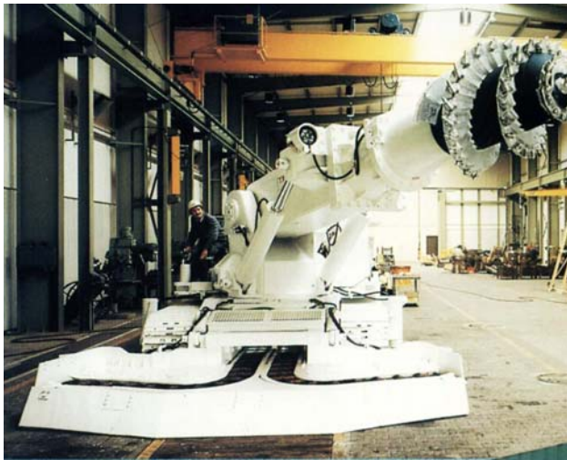
شکل ۳-۱۶-۱۶- ماشین رودهدر با ناوه زنجیری
