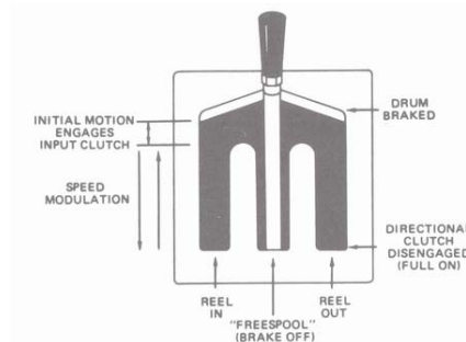
شکل ۶-۹-۷- اهرم کنترل وینچ
