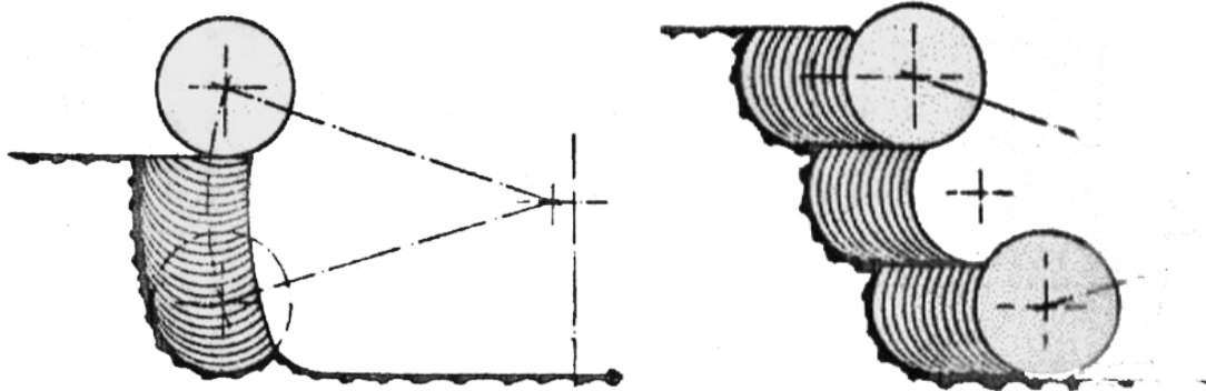
برش پلکانی
