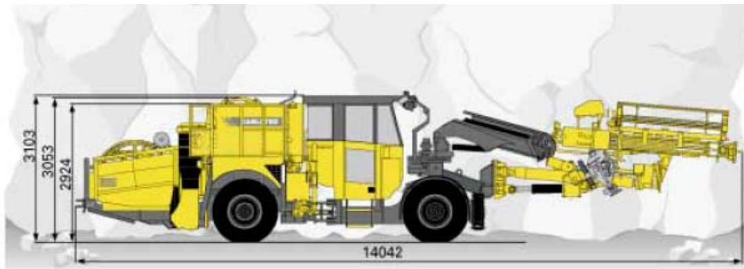
شکل ۳-۲-۴. Cable Bolter
