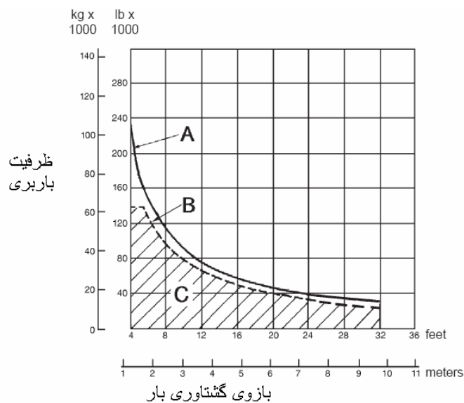
نمودار ۵-۱-۴- نمودار ظرفیت باربری مدل ۵۸۹
