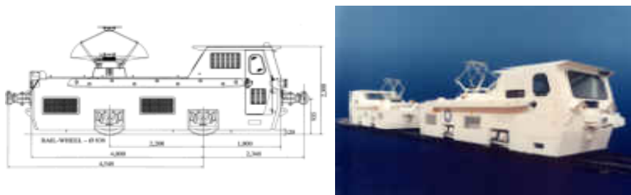
شکل ۳-۱-۳- لکوموتیو با منبع برقی بالاسر
