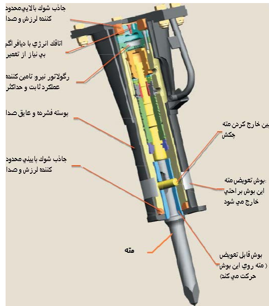
شکل ۲-۱۵-۶- اجزای چکش
