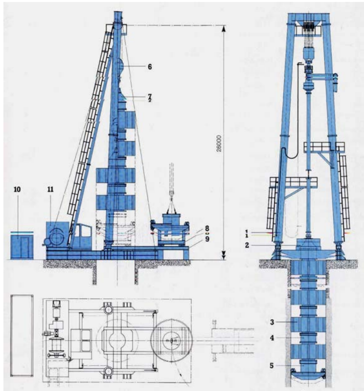
شکل ۳-۱۴-۷. نمای کلی از دکل و تجهیزات داخل چاه ماشین
