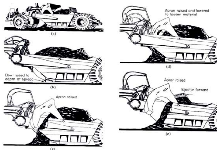
شکل ۳-۶-۲. عملیات تخلیه اسکرپیر
