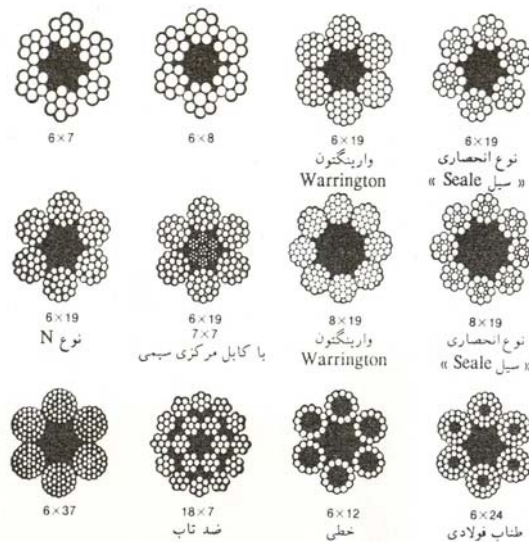
شکل ۶-۵-۳- انواع کابل‌های فولادی
