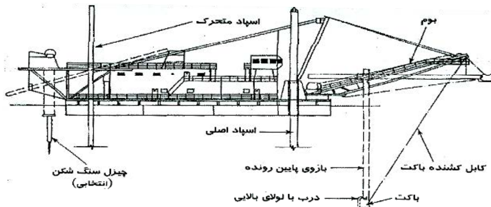
شکل ۵-۸-۱۳- لایروب پیمانانه دار- دیبر
