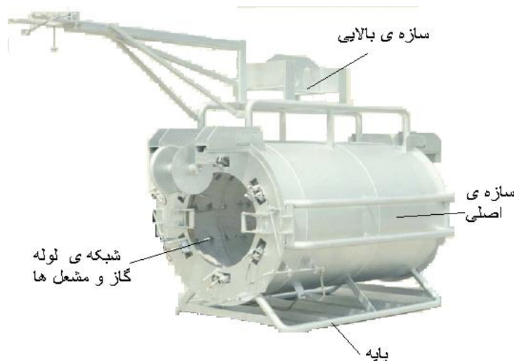
شکل ۳-۳-۵- قسمتهای اصلی پیش گرم کن لوله
