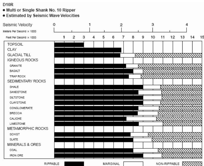
جدول شماره ۲-۳-۴- سرعت موج با توجه به نوع خاک و سنگ برای بولدوزر D10R
