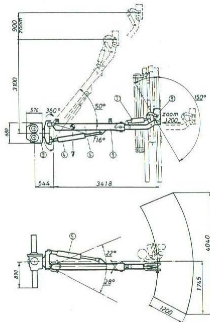
شکل ۳-۲-۸- قسمت‌های مختلف بازو
