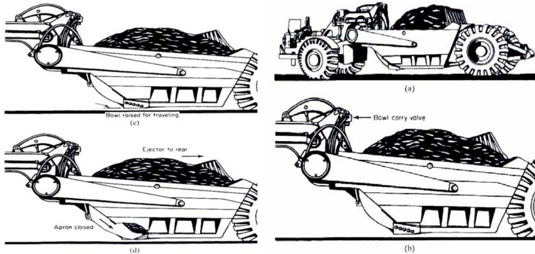
شکل ۲-۶-۲- طریقہ حمل بار توسط اسکرپیر
