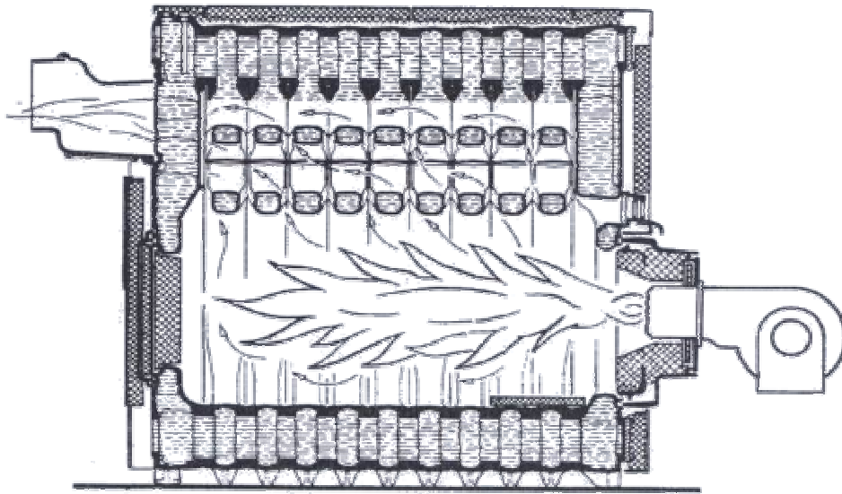
شکل ۴-۷-۱- دیگ چدنی
