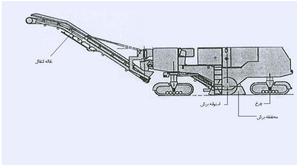
شکل شماره ۲-۱۳-۴- قسمت‌های مختلف ماشین آسفالت تراش
