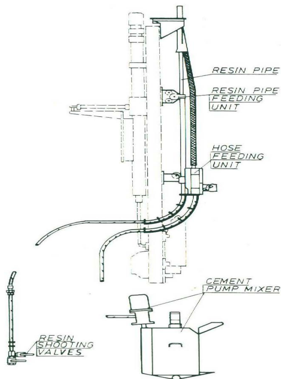
شکل ۳-۲-۷. تغذیه کننده دوغاب
