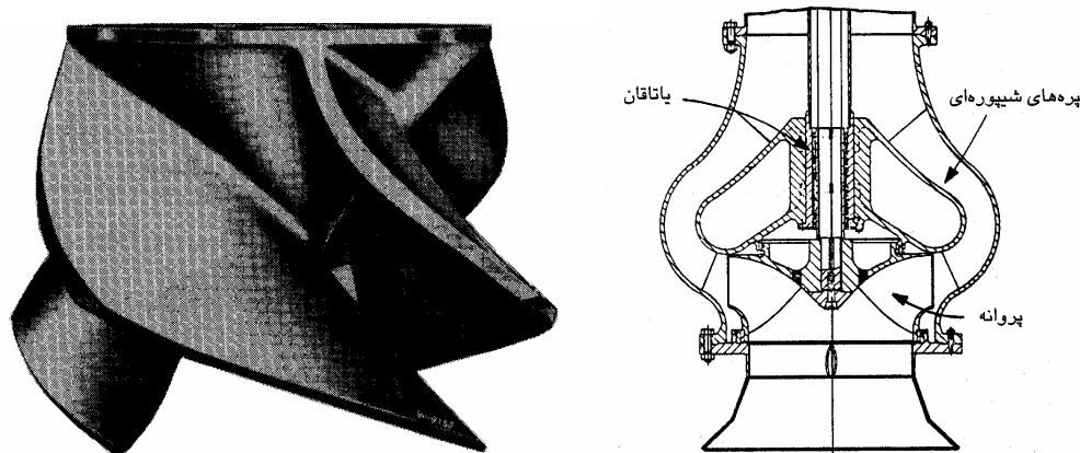
شکل ۶-۱۱-۵- نمایش مقطع و پروانه به کار رفته در پمپ پروانه‌ای جریان مختلط
