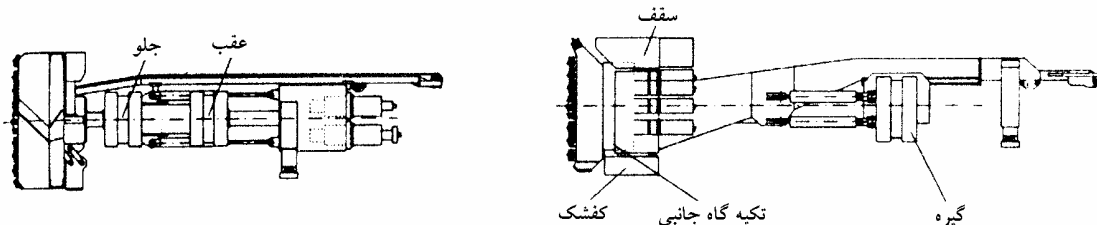
تی بی ام باز دو گیره‌ای
