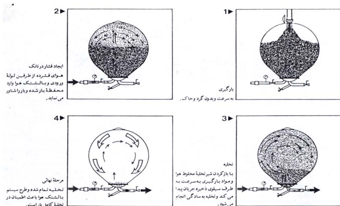
شکل ۴-۱۱-۵- فرایندهای تغذیه و تخلیه بونکر
