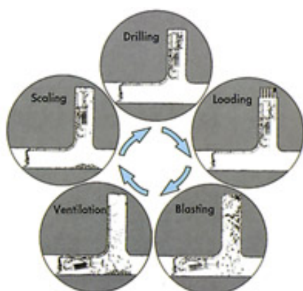
شکل ۶-۱۰-۱- حفاری بالارونده
