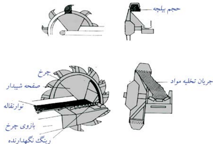
شکل ۳-۳۰-۶- گنجایش چرخ و مسیر تخلیه مواد
