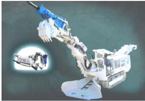
شکل ۳-۱۰-۹- نمایی از ماشینهای چکش هیدرولیکی به همراه سیستم بارگیری
