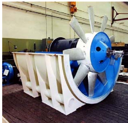
شکل ۶-۱۴-۱-۱- نمایشی از یک بادبزن
