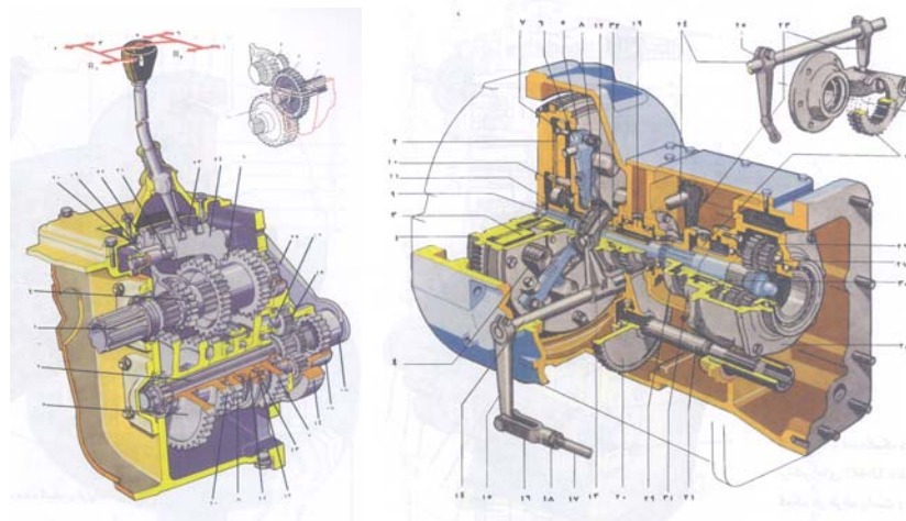
شکل ۶-۱-۸- انواع دنده کمک (سیاره‌ای بدون دنده U600 سیاره‌ای کامل U400)
