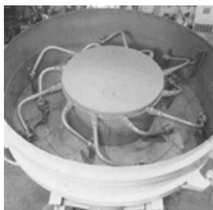
شکل شماره ۴-۳-۹- نمونه میکسر عمودی
