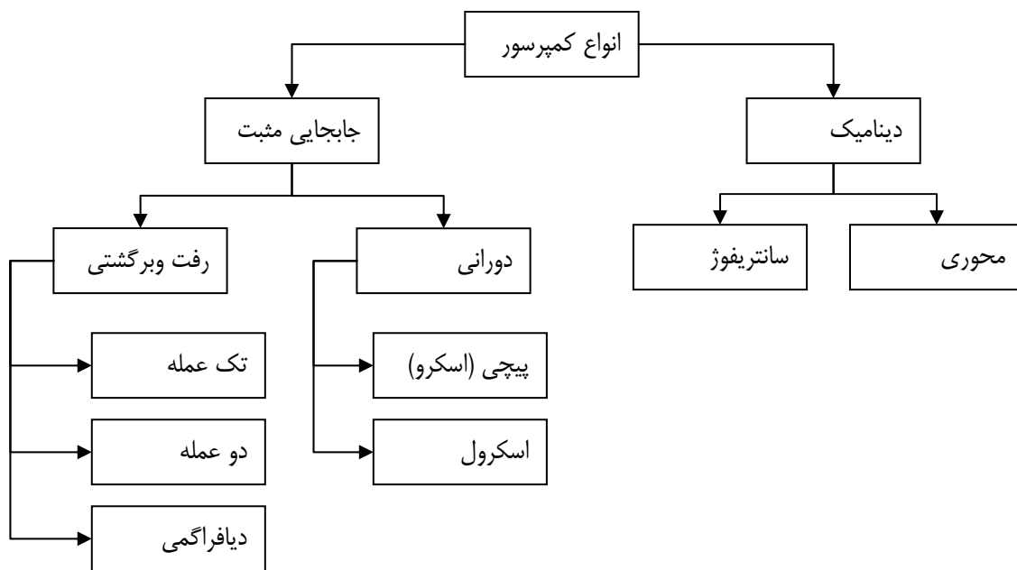
شکل ۶-۱۲-۱- انواع کمپرسور بر حسب نحوه تراکم
