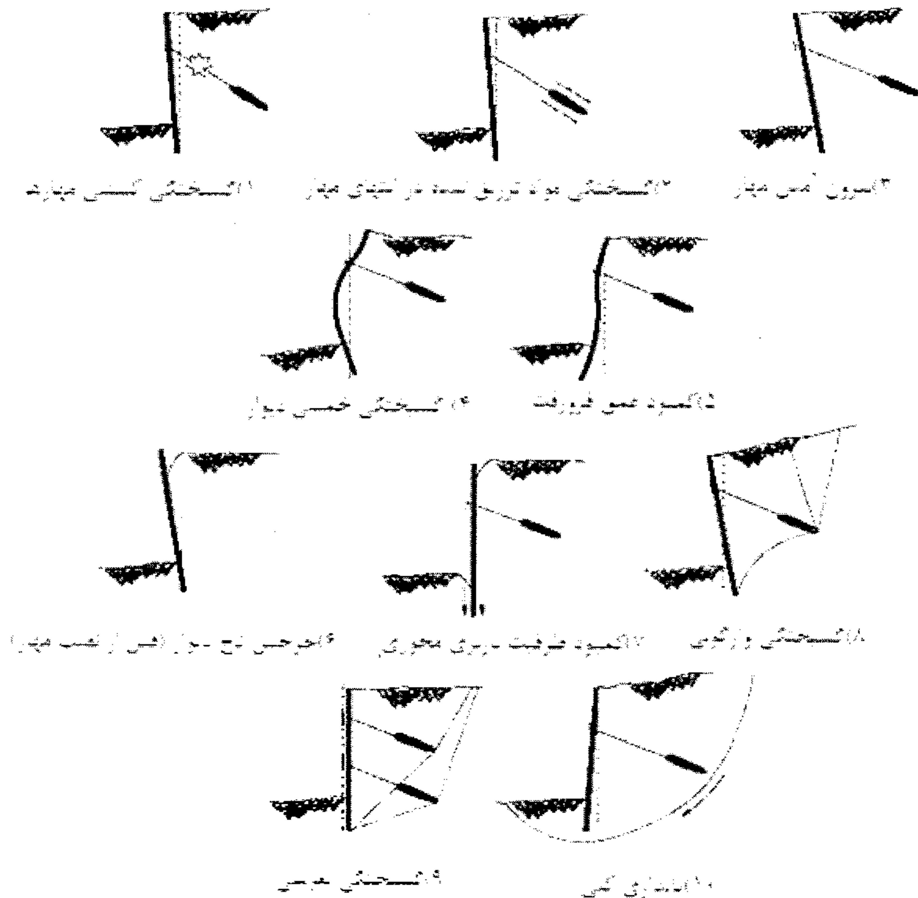
شکل ۷-۵-۱ حالت‌های حدی دیوارهای مهار شده
