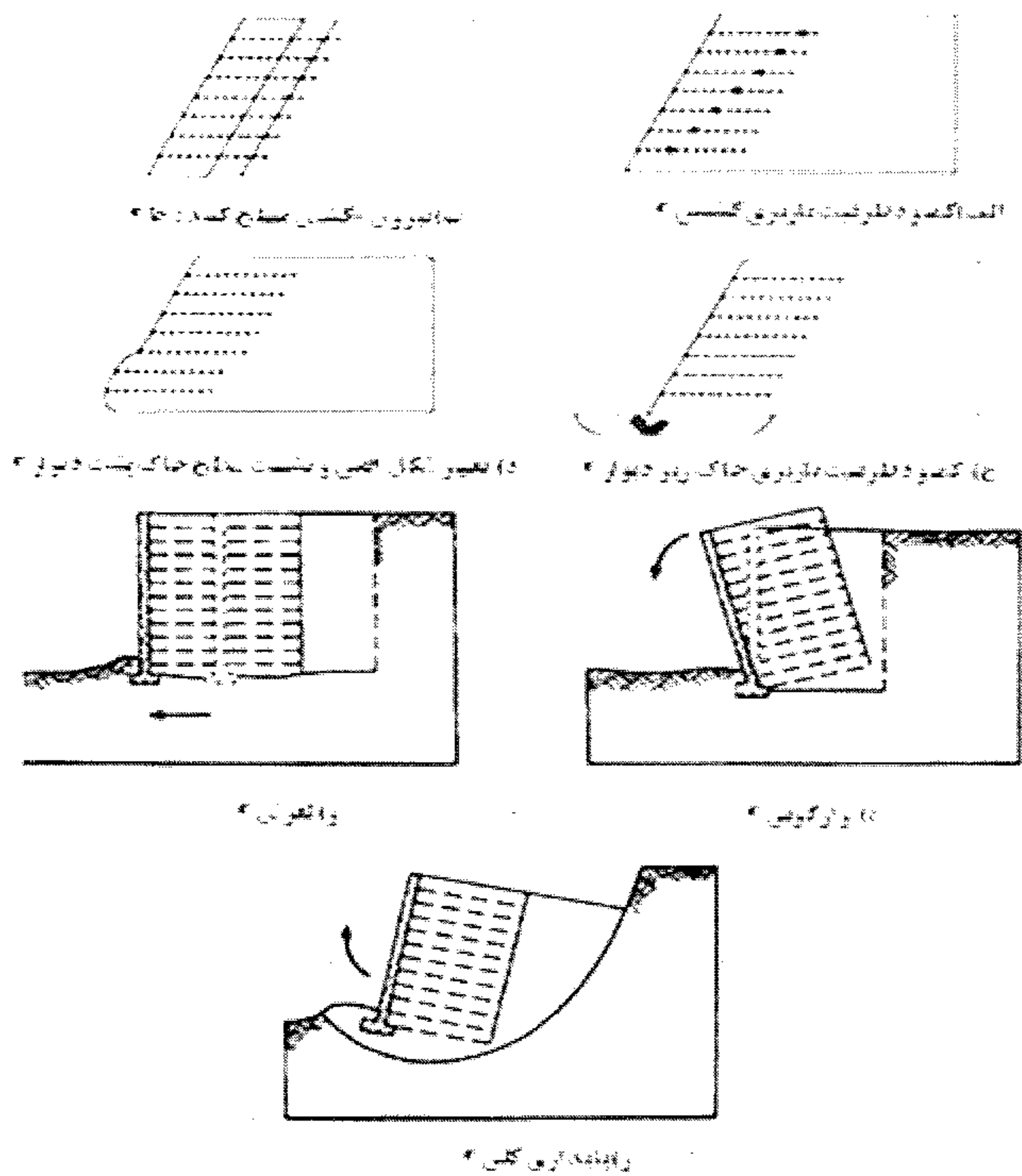
شکل ۷-۵-۲ حالت‌های حدی دیوارهای خاک مسلح
