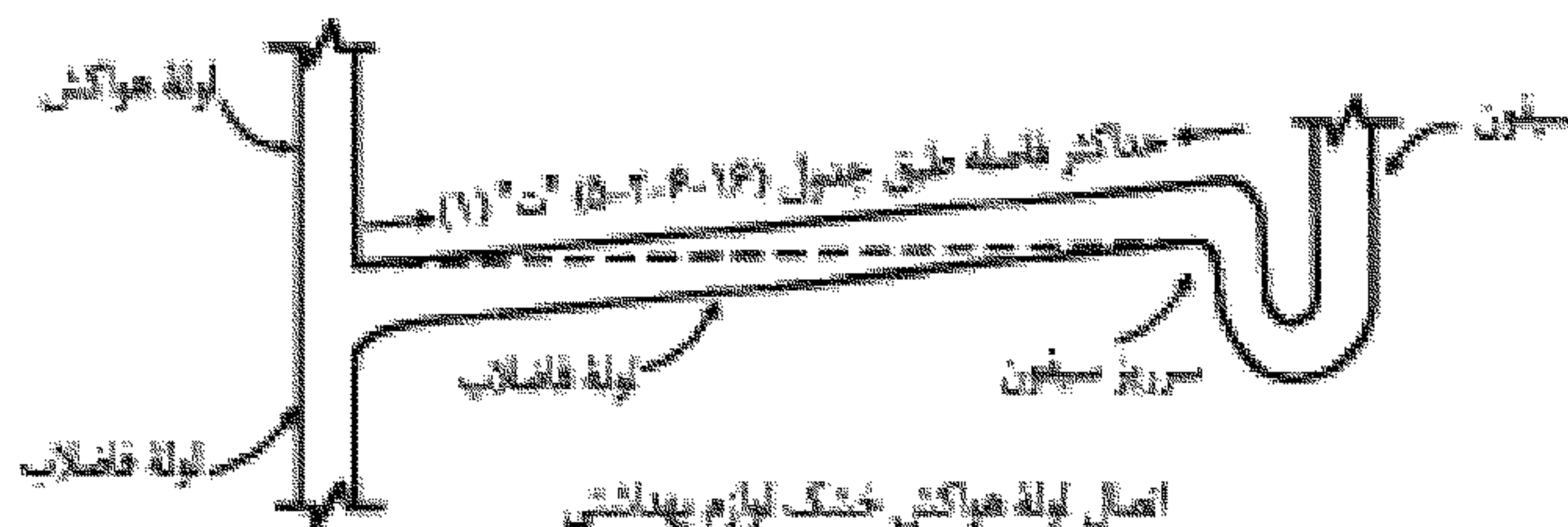
شکل شماره (۵-۲-۶-۱۶) "ت": اتصال لوله هواکش خشک لوازیم بهداشتی
