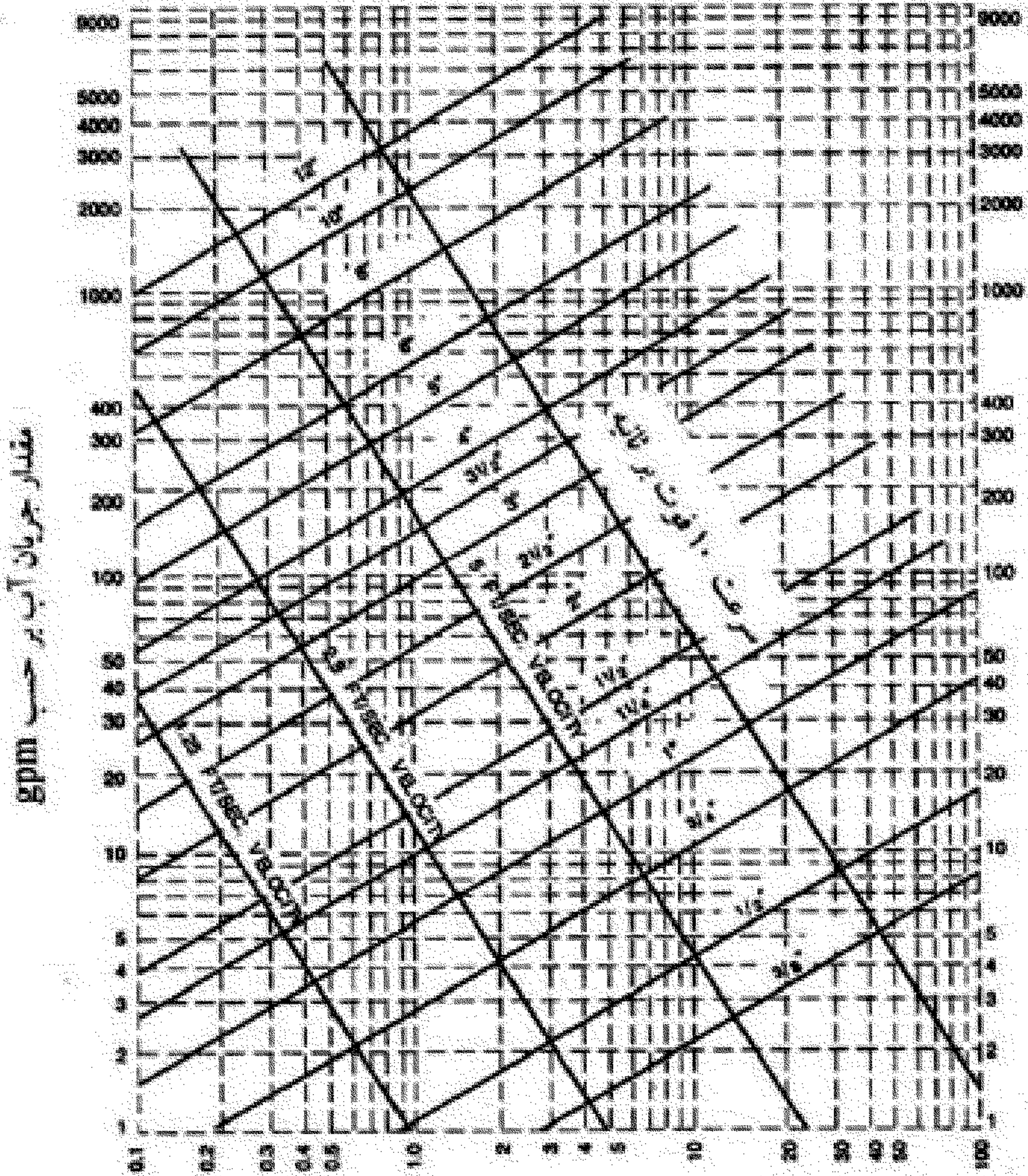
شکل پ ۷-۵-۱ (IP) منحنی اندازه گذاری لوله‌های مسی نوع M از استاندارد ANSI B 88
