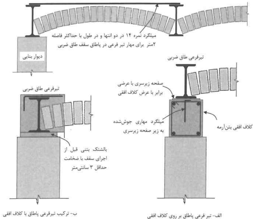
الف- تیر فرعی پاتاق بر روی کلاف افقی
