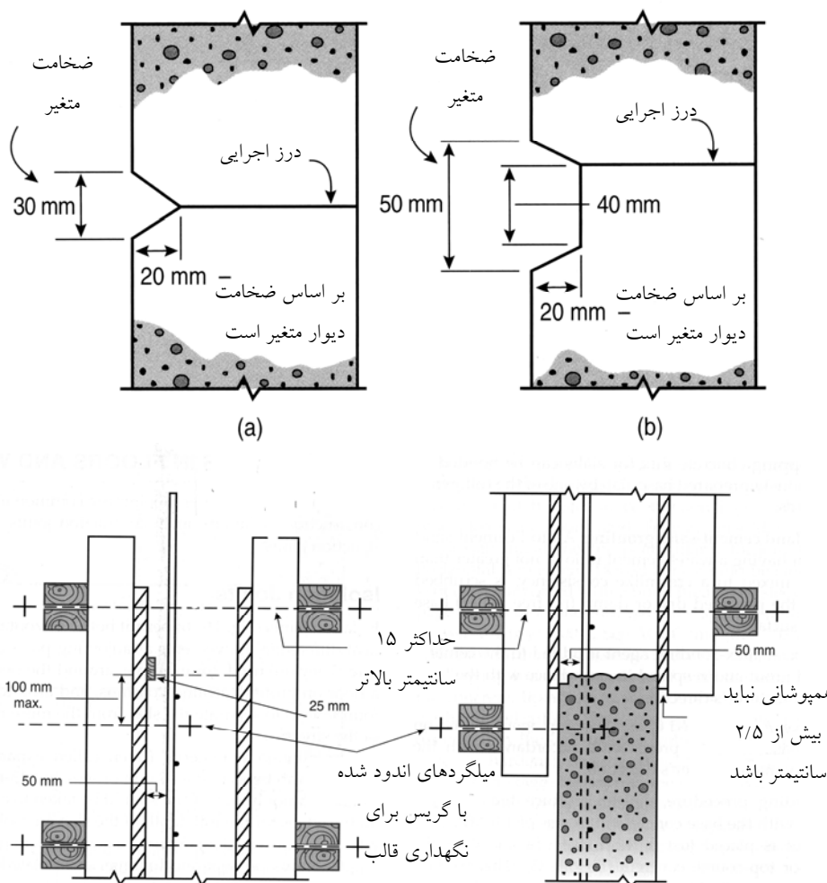
شکل ۱ درز ساخت
